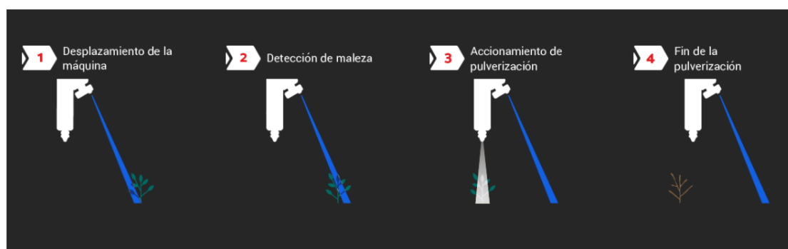
Figura 2: Funcionamiento de un sistema de aplicación selectiva de herbicidas. Fuente: https://weed-it.com.ar/producto/ .
