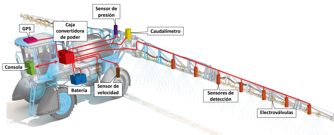
Figura 1: Esquema de componentes de un sistema de aplicaciones selectivas de herbicidas. Adaptado del manual de usuario de WEED-IT Quadro.
