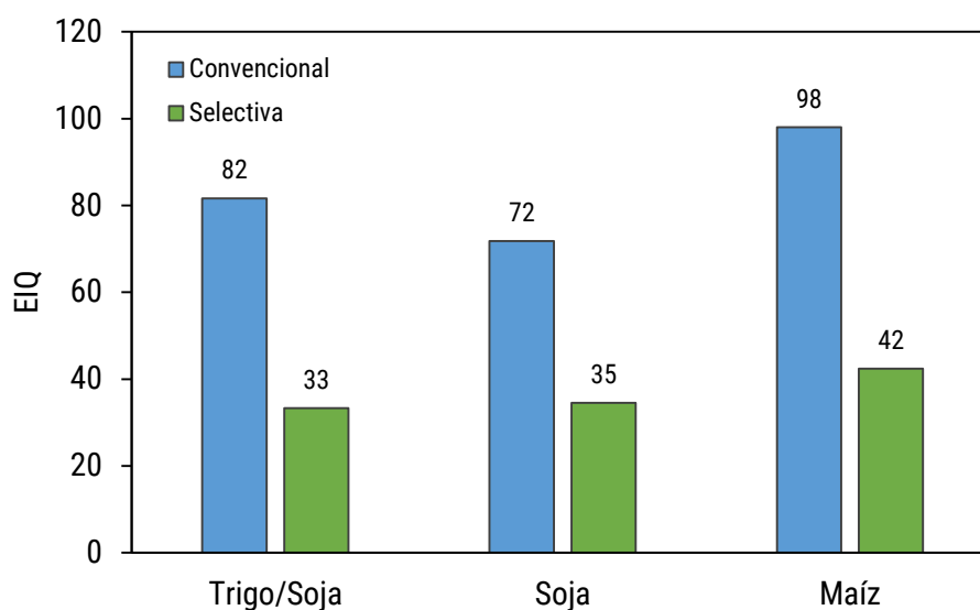
Figura 3. Valores de EIQ en barbechos realizados con aplicaciones en cobertura completa (barras azules) y con un sistema para realizar aplicaciones selectivas de herbicidas (barras verdes) para el doble cultivo Trigo/Soja, y los cultivos de Soja y Maíz.
