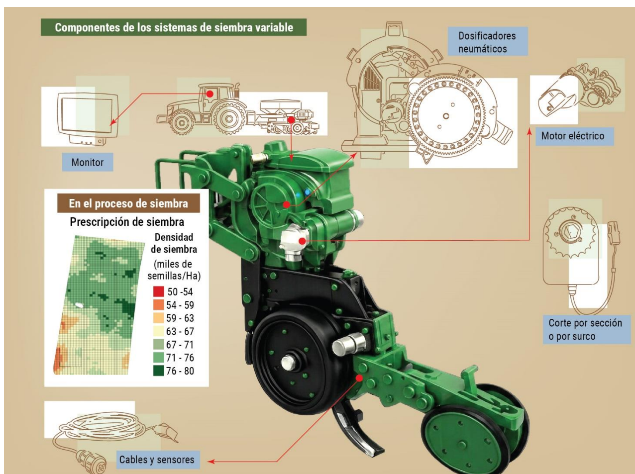
Figura 1. Esquema de componentes que forman parte del sistema para realizar siembra variable.
